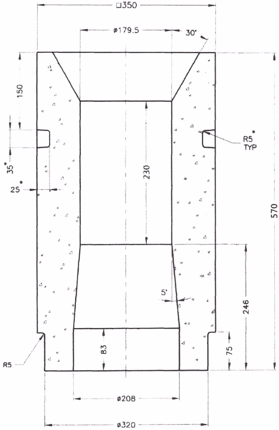
Приложение 3 Чертеж гнездового блока устанавливаемого при первой замене.
