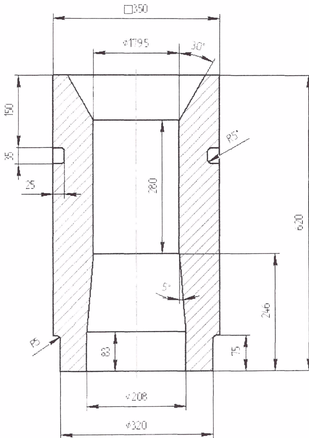
Приложение 2 Чертеж гнездового блока устанавливаемого при изготовлении нового ковша.
