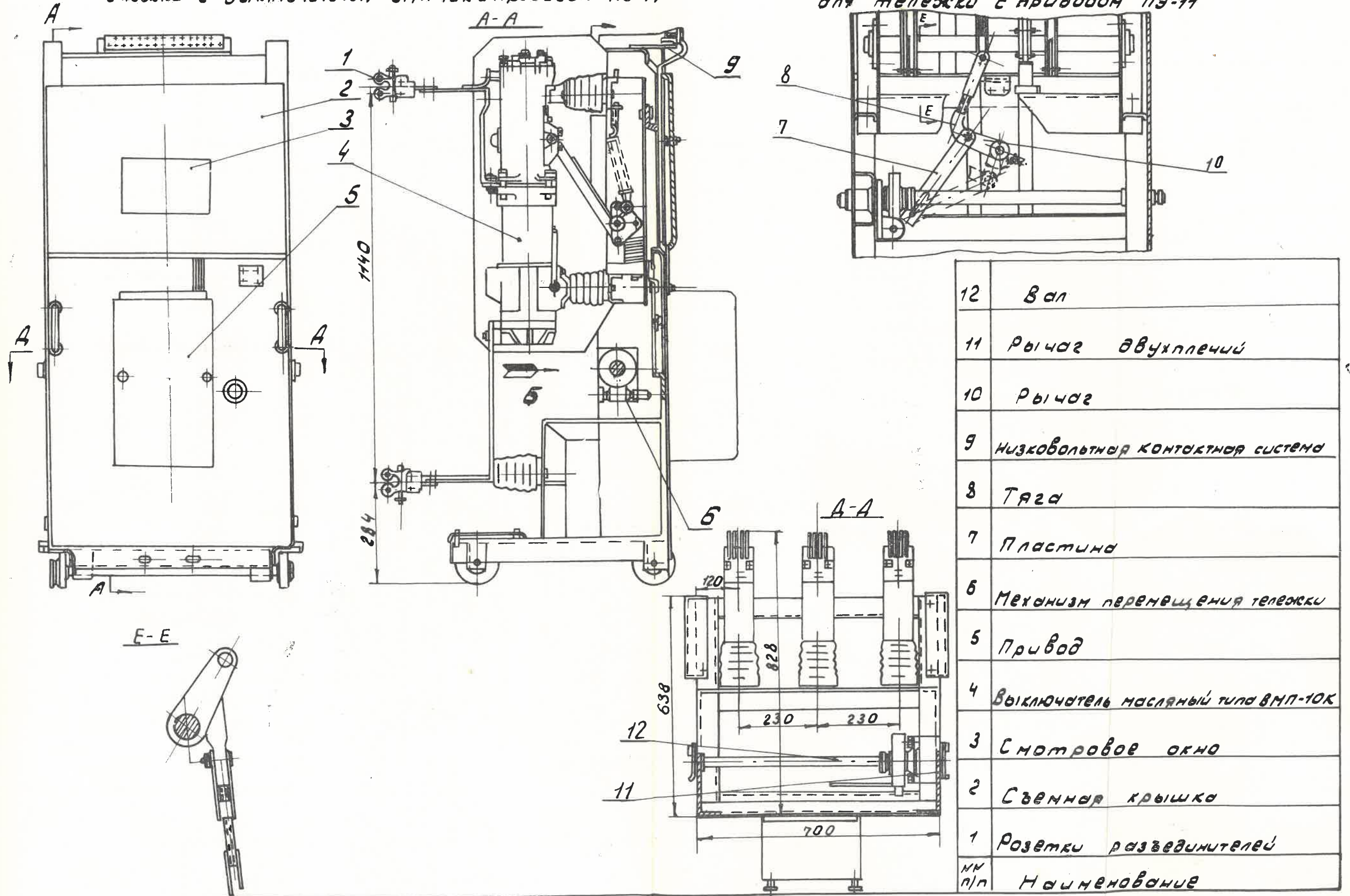
Рис. 4. Тележка с выключателем ВМП-10К и приводом ПЭ-11
